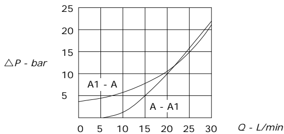
Diagramma perdite di carico Pressure drop curves
